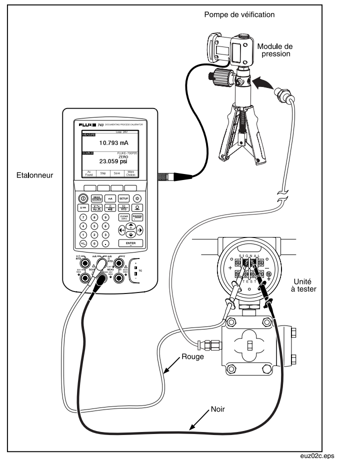
Figure 2. Fonctionnement de la pompe
