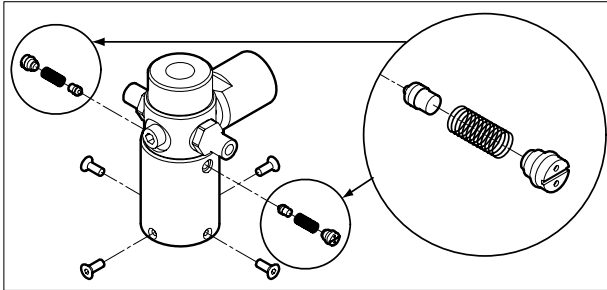
Figure 3. Nettoyage de l'ensemble soupape
