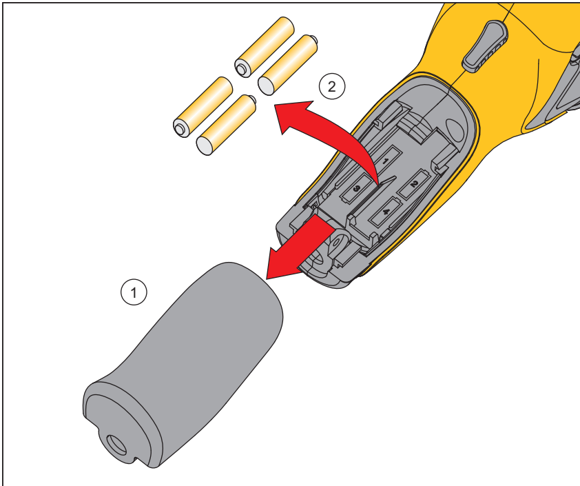
Figur 12. VT02, VT04A Byte av batteri
